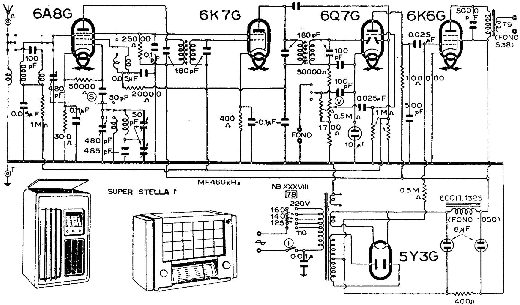
WATT RADIO - MOD. « SUPER STELLA 1 »
